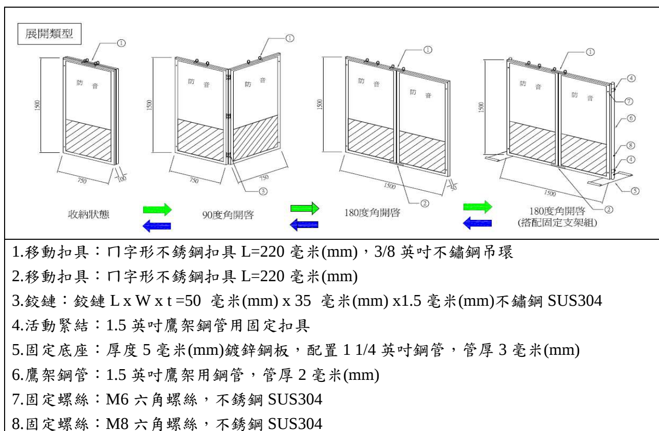
圖 12 移動式隔音屏組裝示意圖
