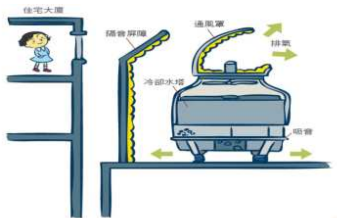
圖 6 冷卻水塔噪音防制方式
